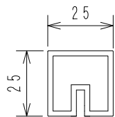
枠詳細 1/2 アルミ押出型材
