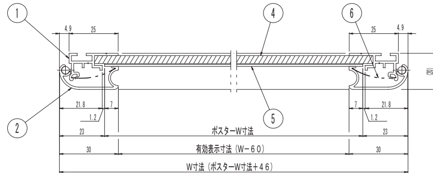
断面 B-B (S=1/1)
