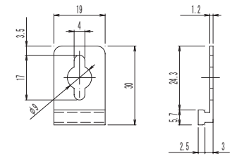
スライド式用金具 (S=1/1)
